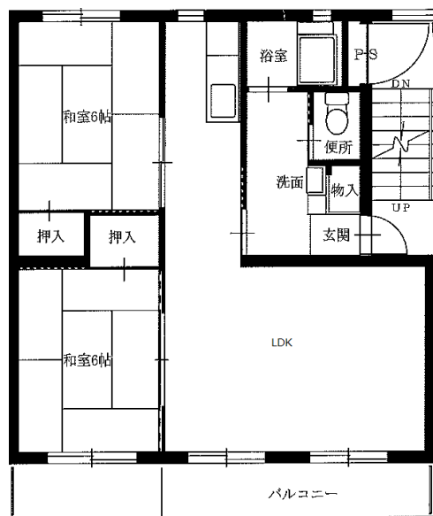
2LDK-B(3-22・13-32・13-44)
